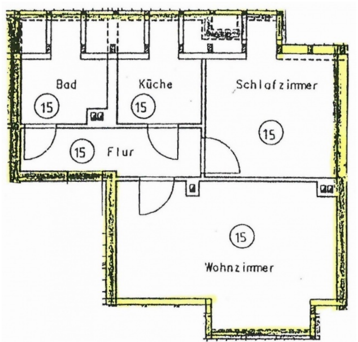
Grundriss
